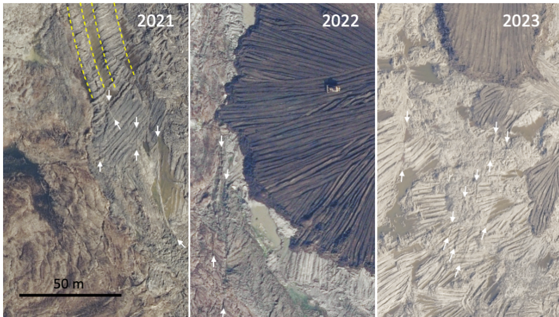
Figur 5. Udsnit af forårs-ortofoto fra den vestlige del af den deponerede jord, som viser sprækkedvikling i hhv. 2021, 2022 og 2023. Sprækkerne er markeret med hvide pile ved start og slut. De stiplede gule streger viser et såkaldt "horst og graben system", der indikerer øst-vest vandret bevægelse. Se Figur 4 for placering.
