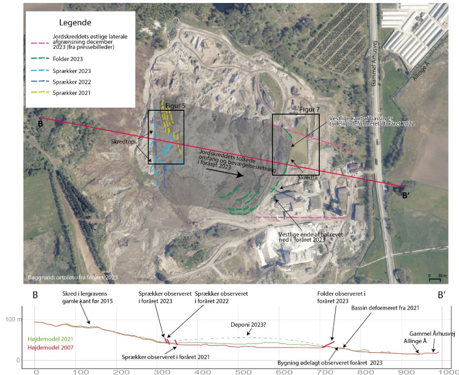
Figur 4. Ortofoto fra foråret 2023 med kortlagte skredstrukturer fra 2021, 2022 og 2023 vist. Desuden er jordskreddets omfang i foråret 2023 vist med grå skygge. Strukturerne viser, at jordskredet har været i bevægelse i siden foråret 2021. De sorte bokse viser udsnit, som ses i Figur 5 og 7. Profilet langs B-B' linjen viser topografien i 2007 samt 2021 langs den røde linje på kortet. Desuden vises, hvor der er observeret sprækker og folder.
