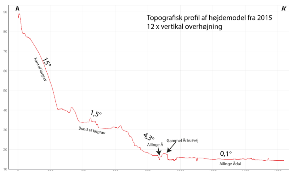
Figur 2. Morfologi i lergravnen i 2015 før deponiet starter. Udglattede 10 m højdekurver er vist oven på en farvelagt højdemodel med skyggelægning. Deponiets og jordskreddets omfang i foråret 2023 er vist med stiplede linjer. Det 12 gange overhøjede topografiske profil nederst viser landskabets hældning langs linjen A-A' på kortet i 2015, strækkende sig fra toppen af lergravnen, ned igennem området, hvor deponiet senere bygges op og ud igennem ådalen.
