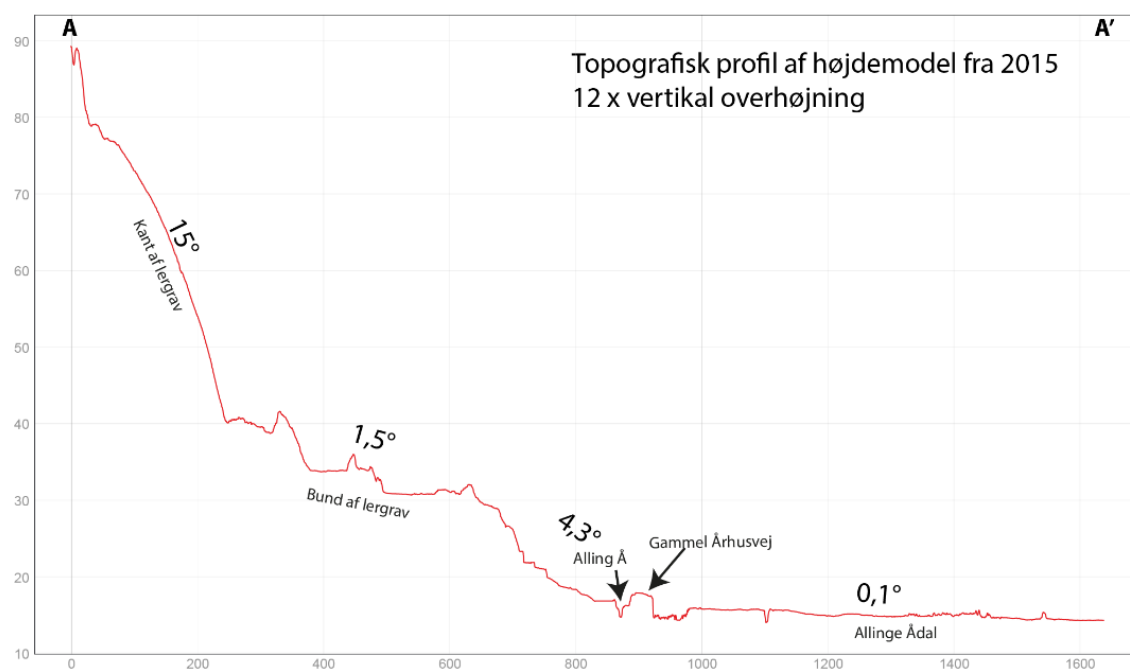
Figur 2. Morfologi i lergraven i 2015. Udglattede 10 m højdekurver er vist oven på en farvelagt højdemodel med skyggelægning. Blå farver ved Alling Å er omkring 15 m over havniveau og rødlige farver vest for lergraven er omkring 90 m over havniveau. Deponiets og jordskreddets omfang i foråret 2023 er vist med stiplede linjer. Det 12 gange overhøjede topografiske profil nederst viser landskabets hældning langs linjen A-A' på kortet i 2015, strækkende sig fra toppen af lergraven, ned igennem området, hvor deponiet senere bygges op og ud igennem ådalen.
