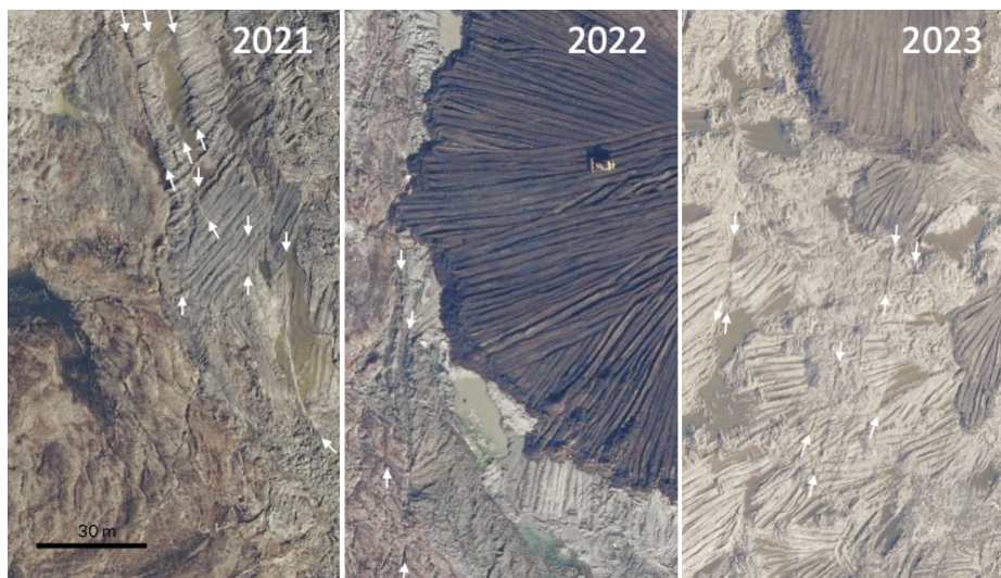
Figur 5: Udsnit af forårs-ortofoto fra den vestlige del af den deponerede jord, som viser sprækkeudvikling i hhv. 2021, 2022 og 2023. Sprækkerne er markeret med hvide pile ved start og slut. Se Figur 4 for placering.
