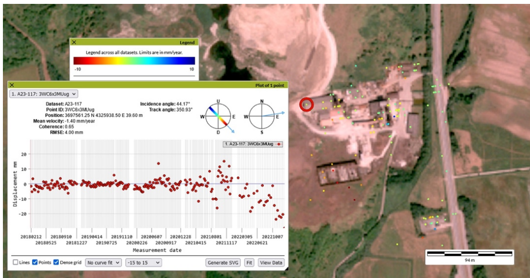
Figur 6. Udsnit fra European Ground Motion Service (EGMS) webportalen, som viser terrænbevægelser på bygningerne ved Nordic Waste. Målingerne i nedre venstre hjørne viser et tydeligt skift i InSAR-dataserierne, som indikerer en begyndende påvirkning af det bebyggede område i første halvdel af 2021.
