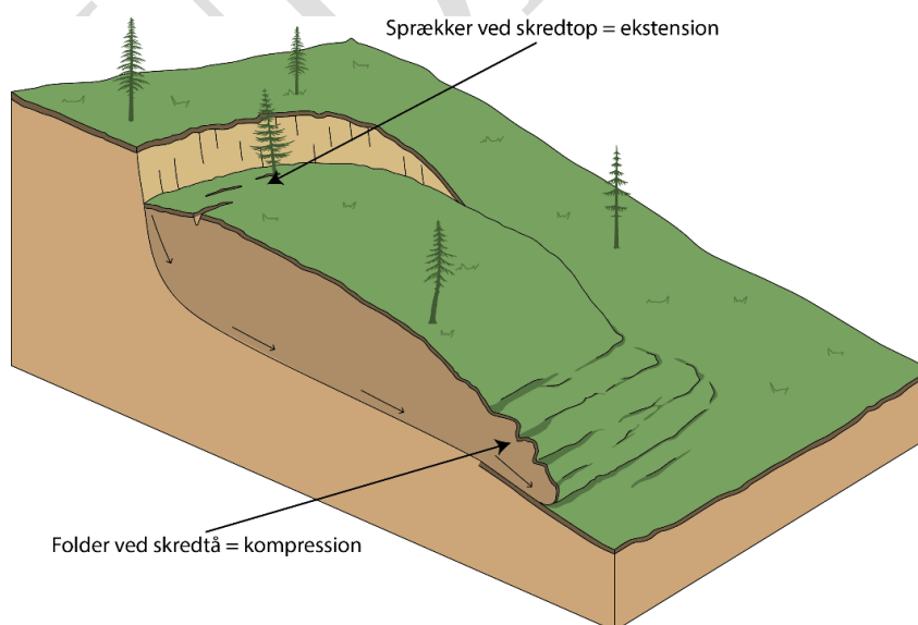
Figur 1. Blokdigram af et generaliseret landskred med overordnet nomenklatur. Pilene viser skreddets bevægelse.
