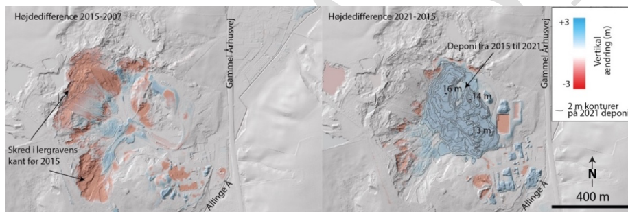
Figur 3. Differentialhøjdemodeller for området ved Nordic Waste. Til venstre 2007–2015 og til højre 2015–2021. Blå farver betyder at terrænet er blevet højere, og røde farver at det er blevet lavere. På figuren til højre er indtegnet konturer for hver 2 m samt enkelte maksimumhøjder for den deponerede jord i 2021. Volumen af materialet deponeret fra 2015 til 2021 (det konturerede område) svarer til 0,8 millioner m^3 .
