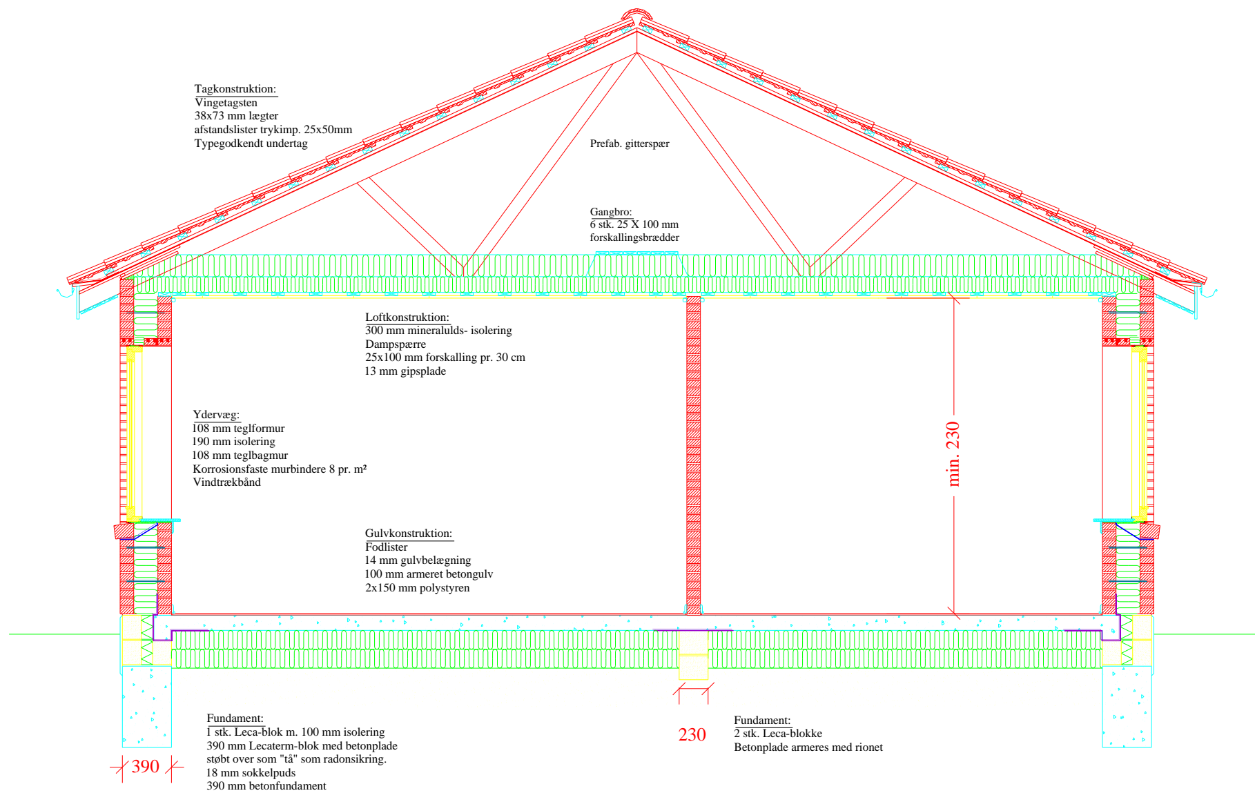
Tværsnit 1:50
